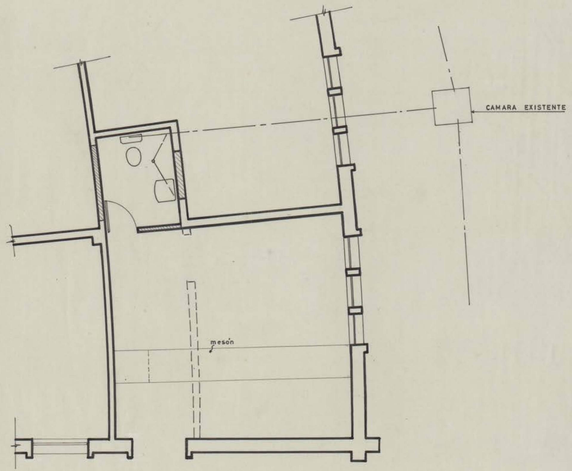
PLANTA Esc. 1: 50
