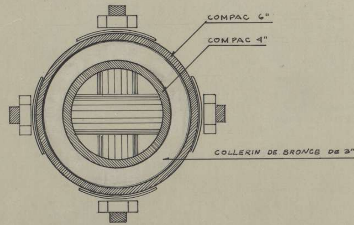
CORTE B-B
