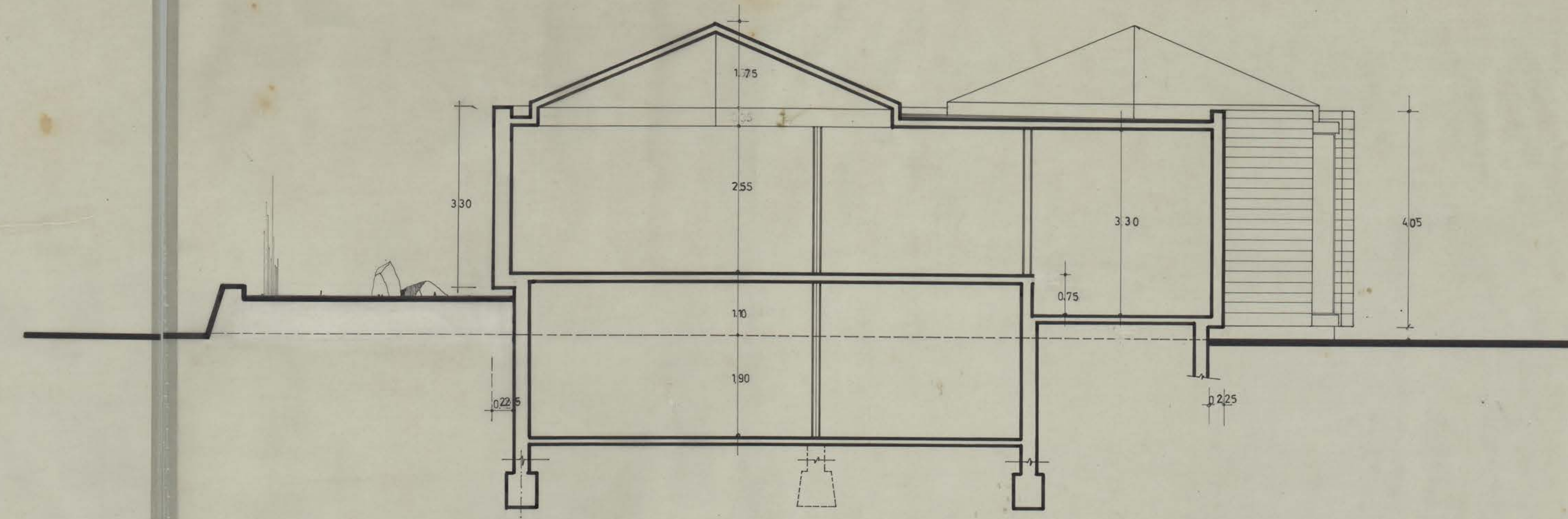
CORTE SALAS DE EXPOSICION (VER LAMINA 9 CORTE ESC. 1/20)
