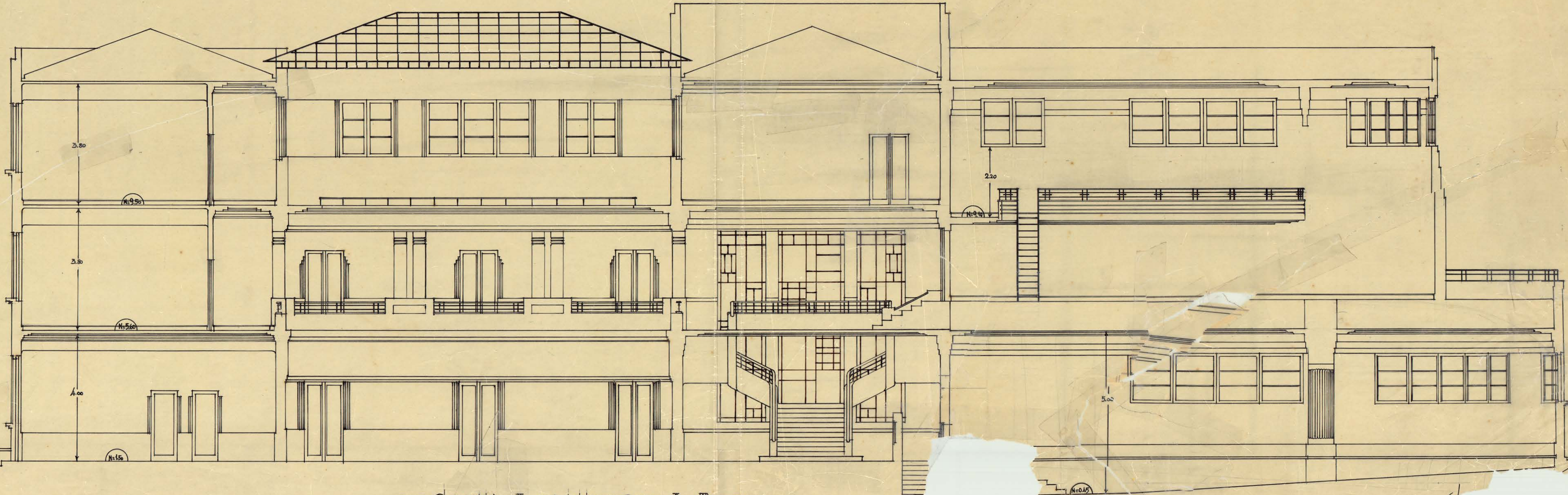
CORTE LONGITUDINAL A-B
