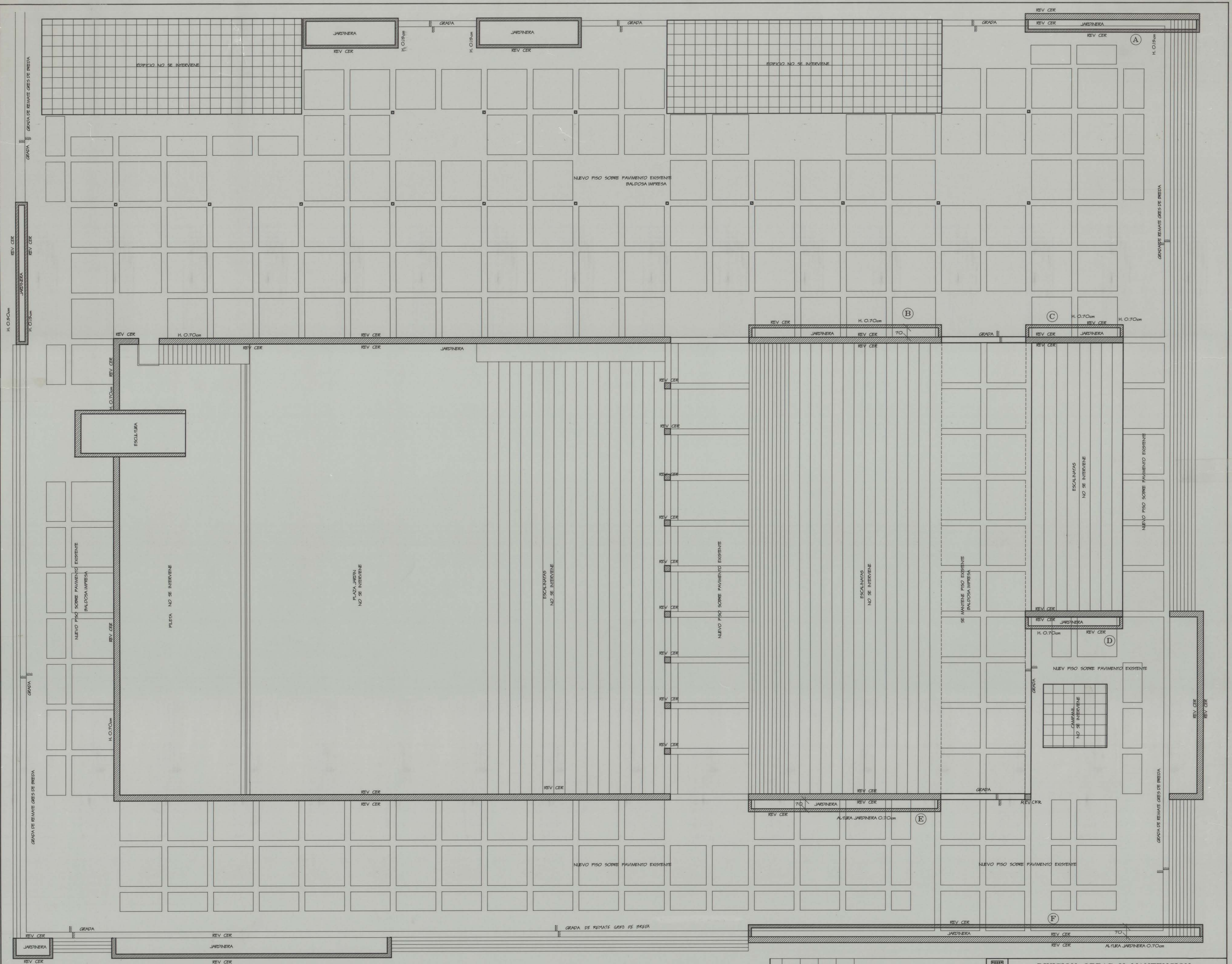
PLANTA DE PAVIMENTOS PLAZA FORO
