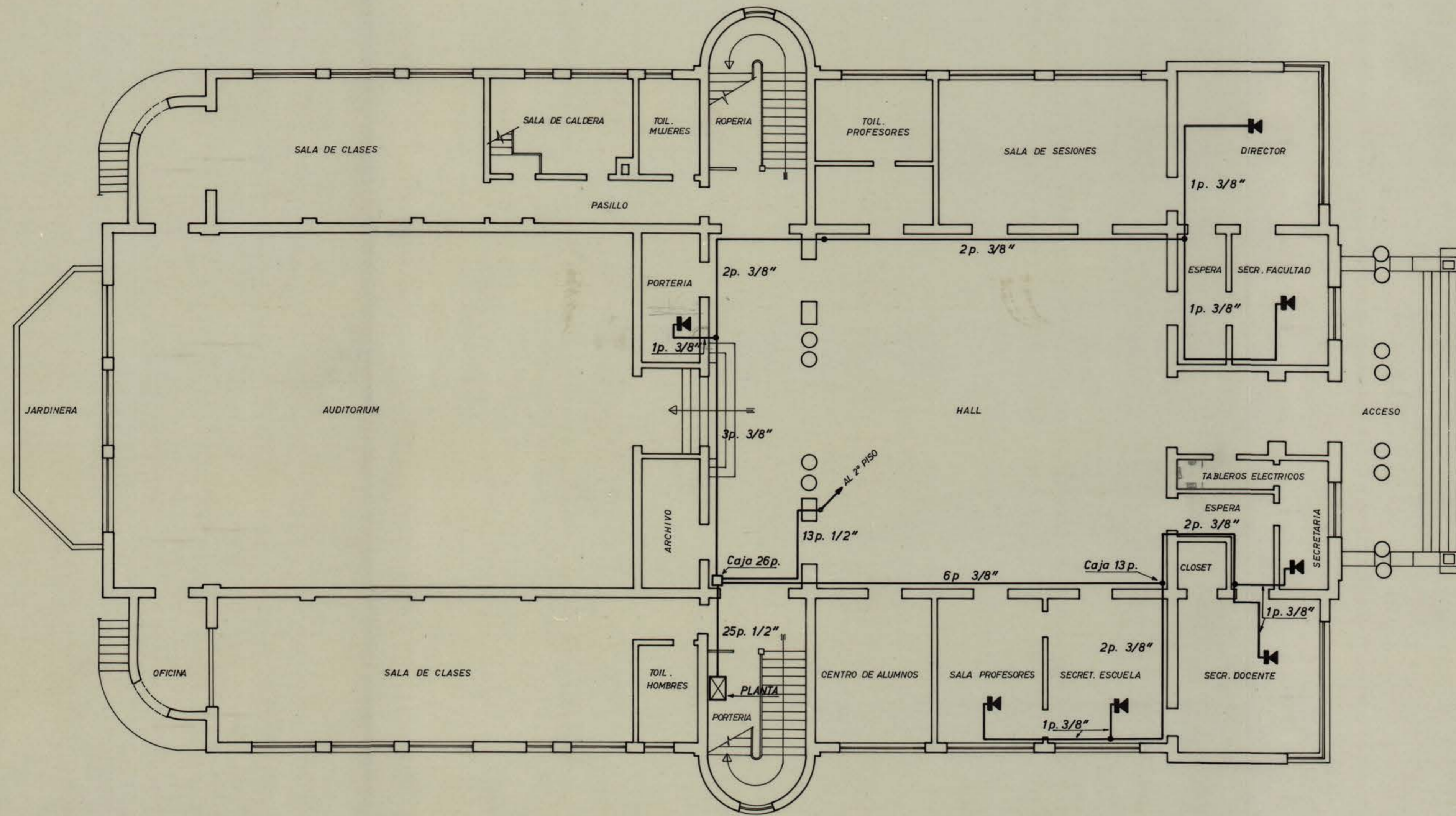
PLANTA DEL PRIMER PISO ESC. 1:100
