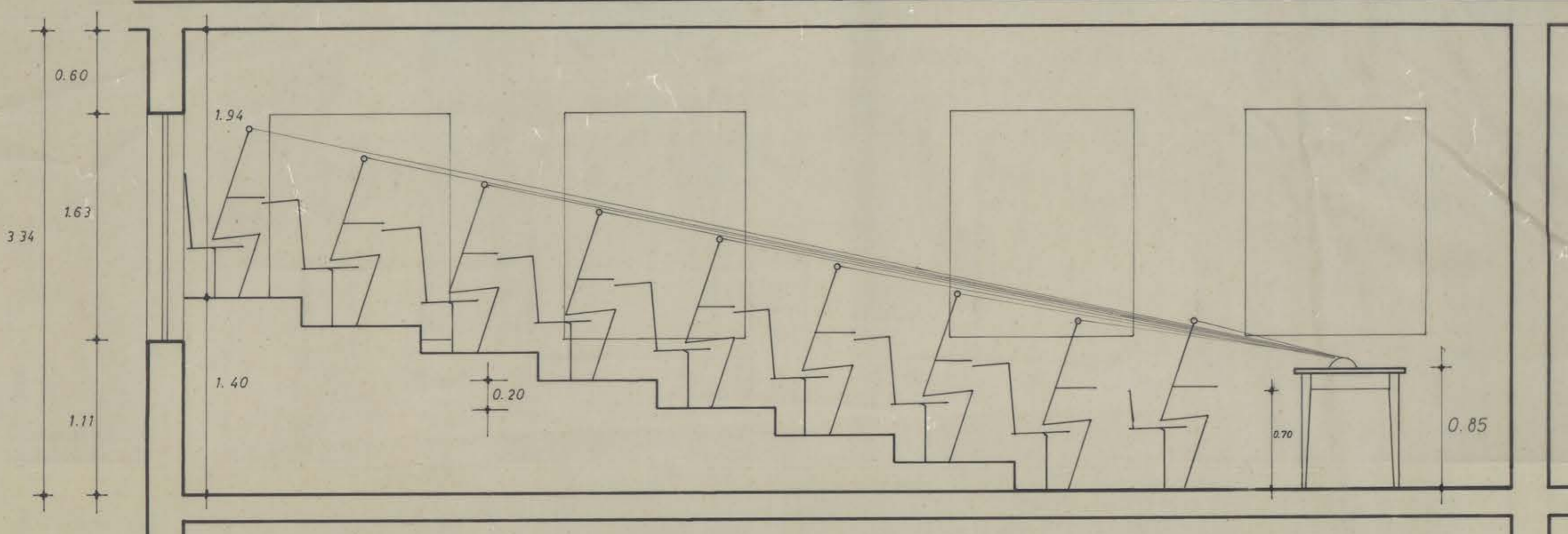
ELEVACION ESC. 1 : 25
