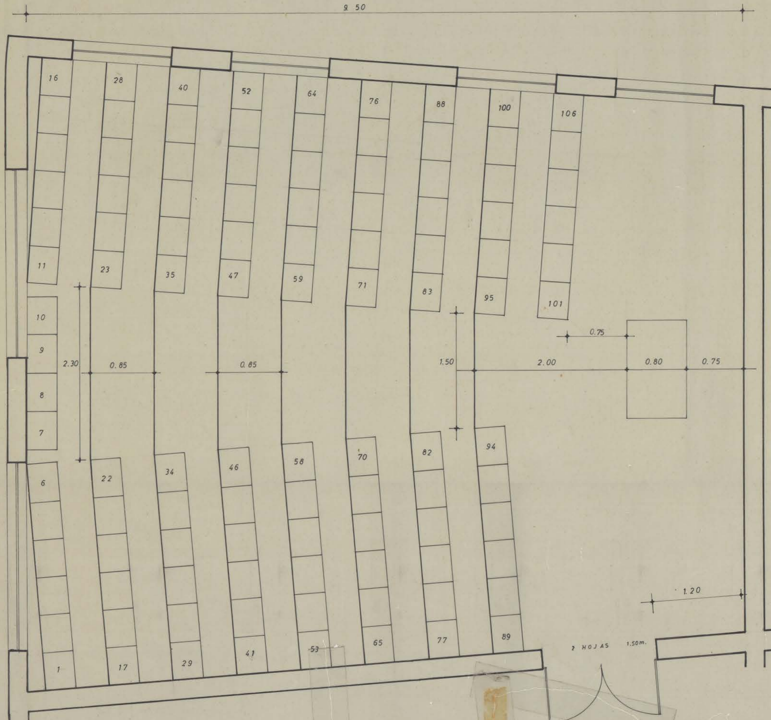
PLANTA ESC. 1 : 25
