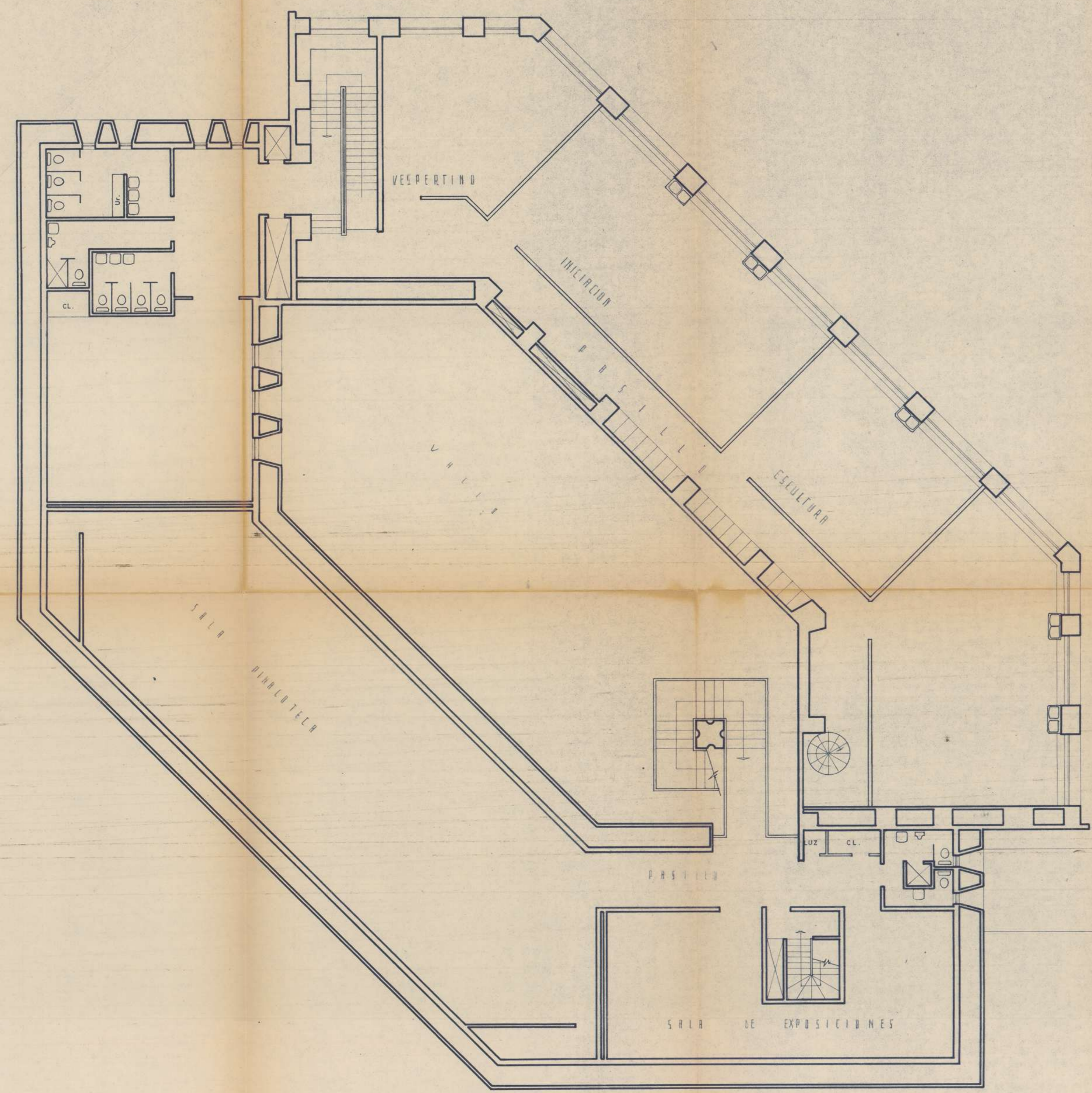
PLANTA SEGUNDO PISO ESC. 1:100
