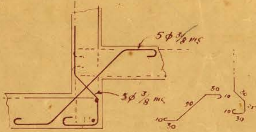
Sec. a-a Esc. 1:20
