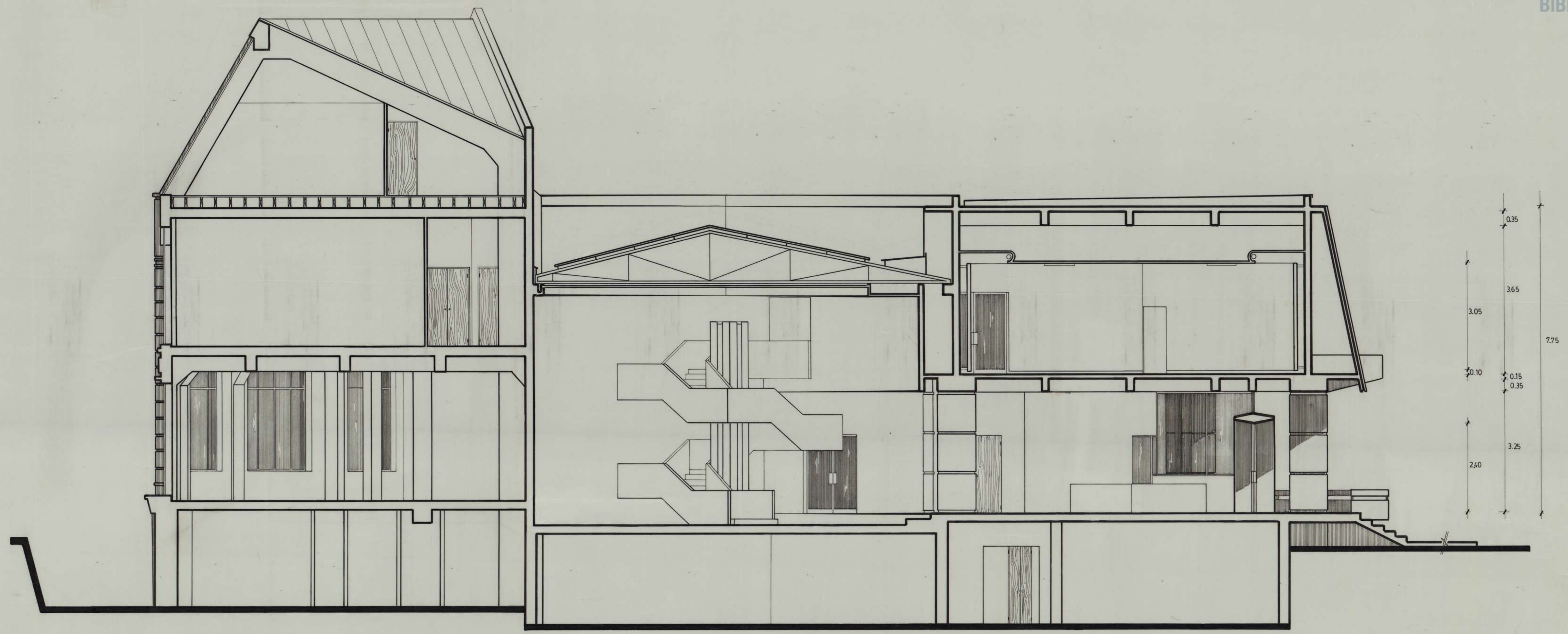
CORTE A-A ESCALA 1:50
