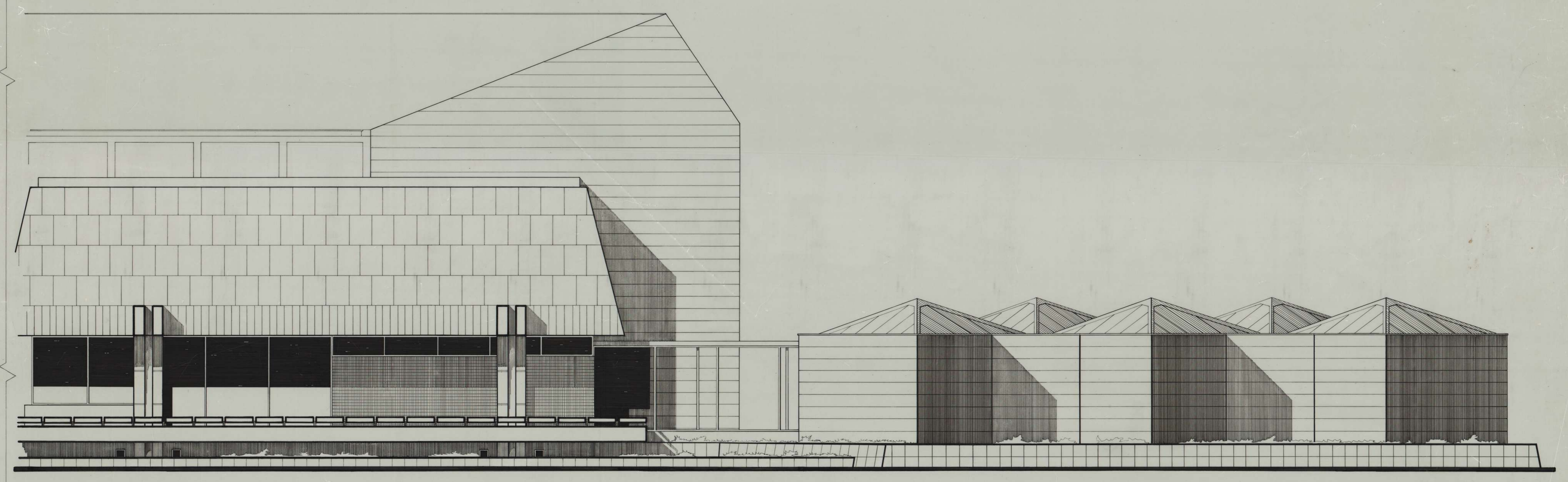
CASA DEL ARTE UNIVERSIDAD DE CONCEPCION ARQUITECTOS ALEJANDRO RODRIGUEZ OSVALDO CACERES ELEVACION LATERAL ESCALA 1:50
