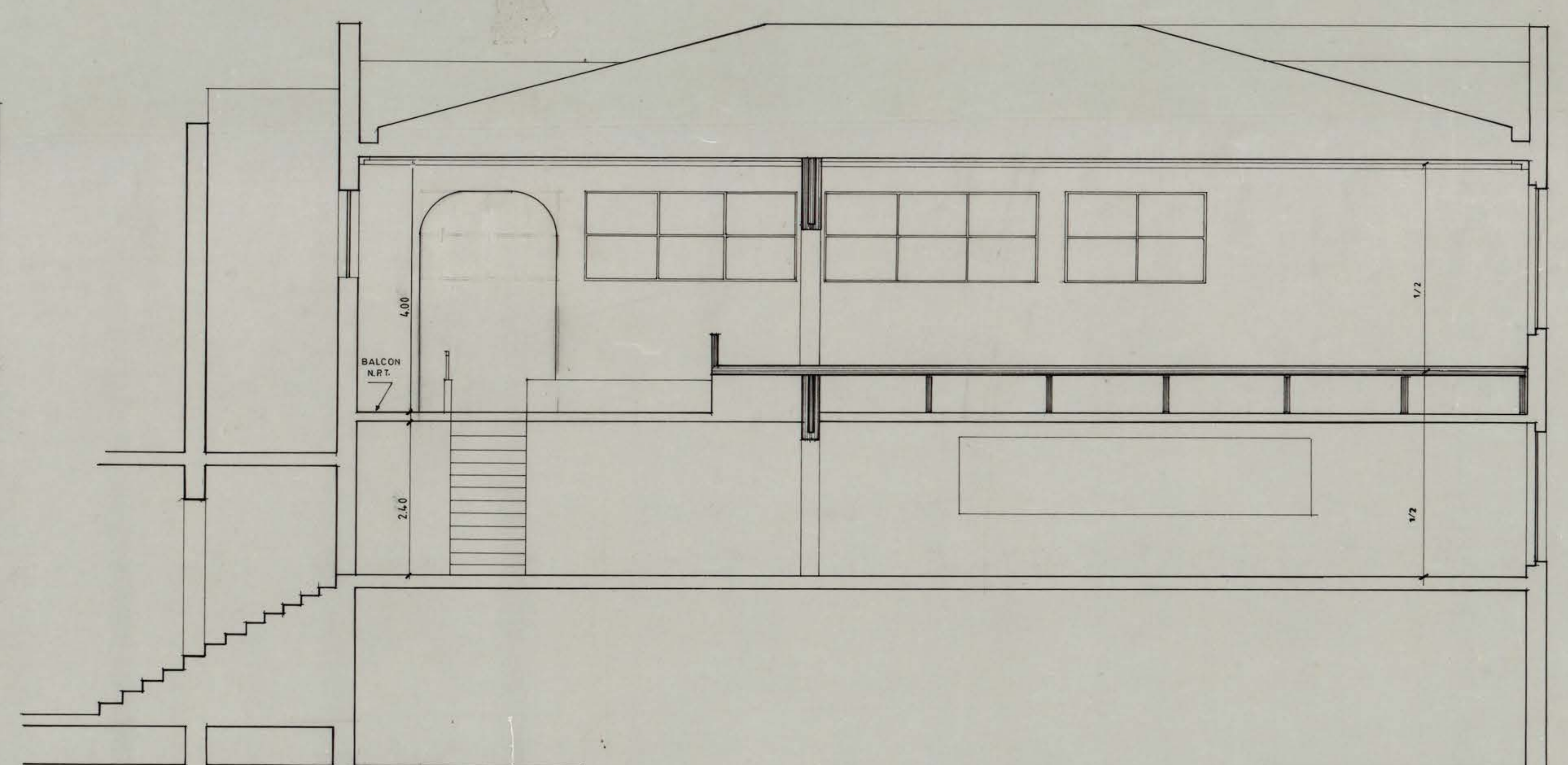
CORTE C-D ESC: 1:50
