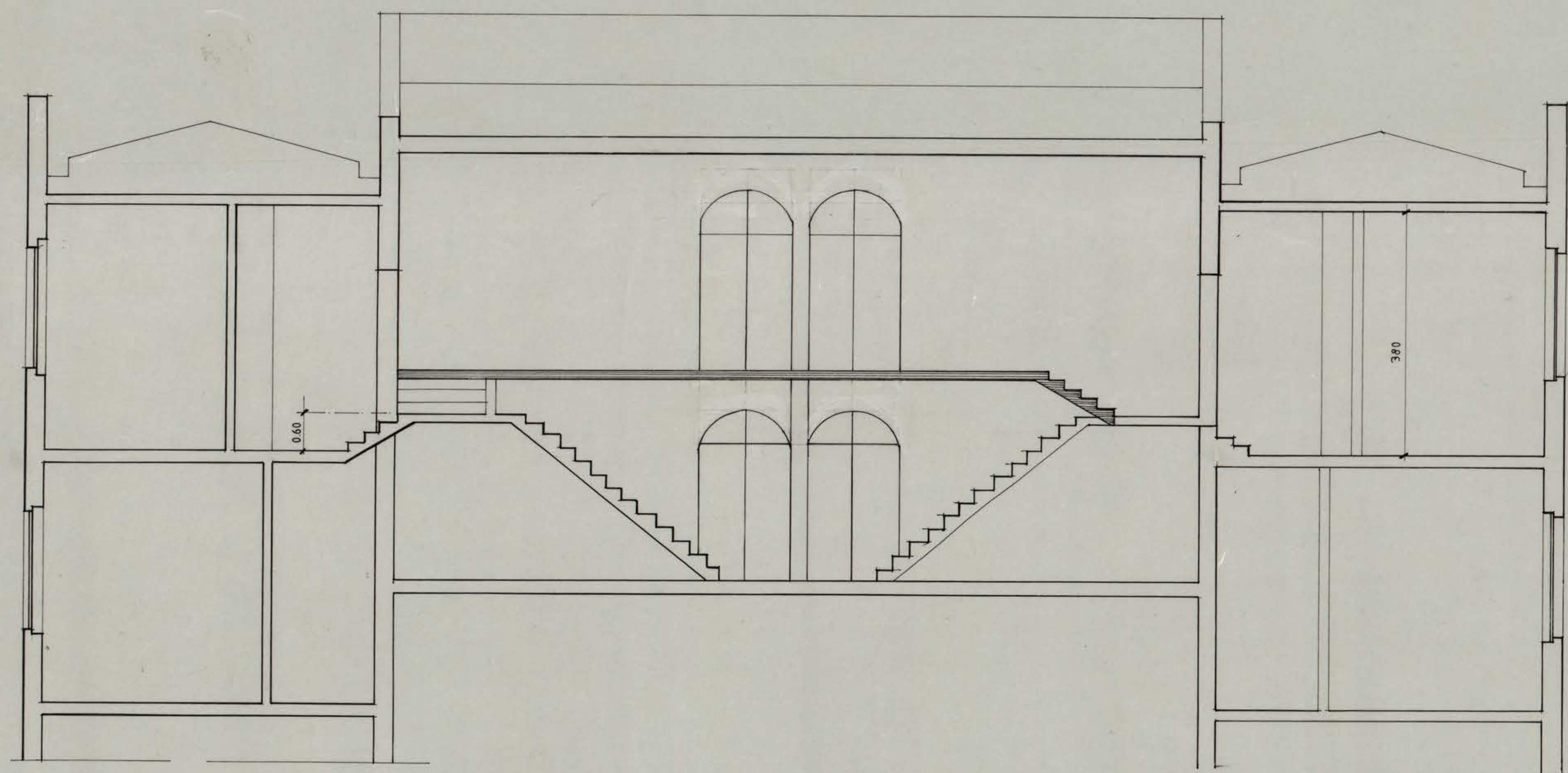
CORTE A-B ESC: 1:50
