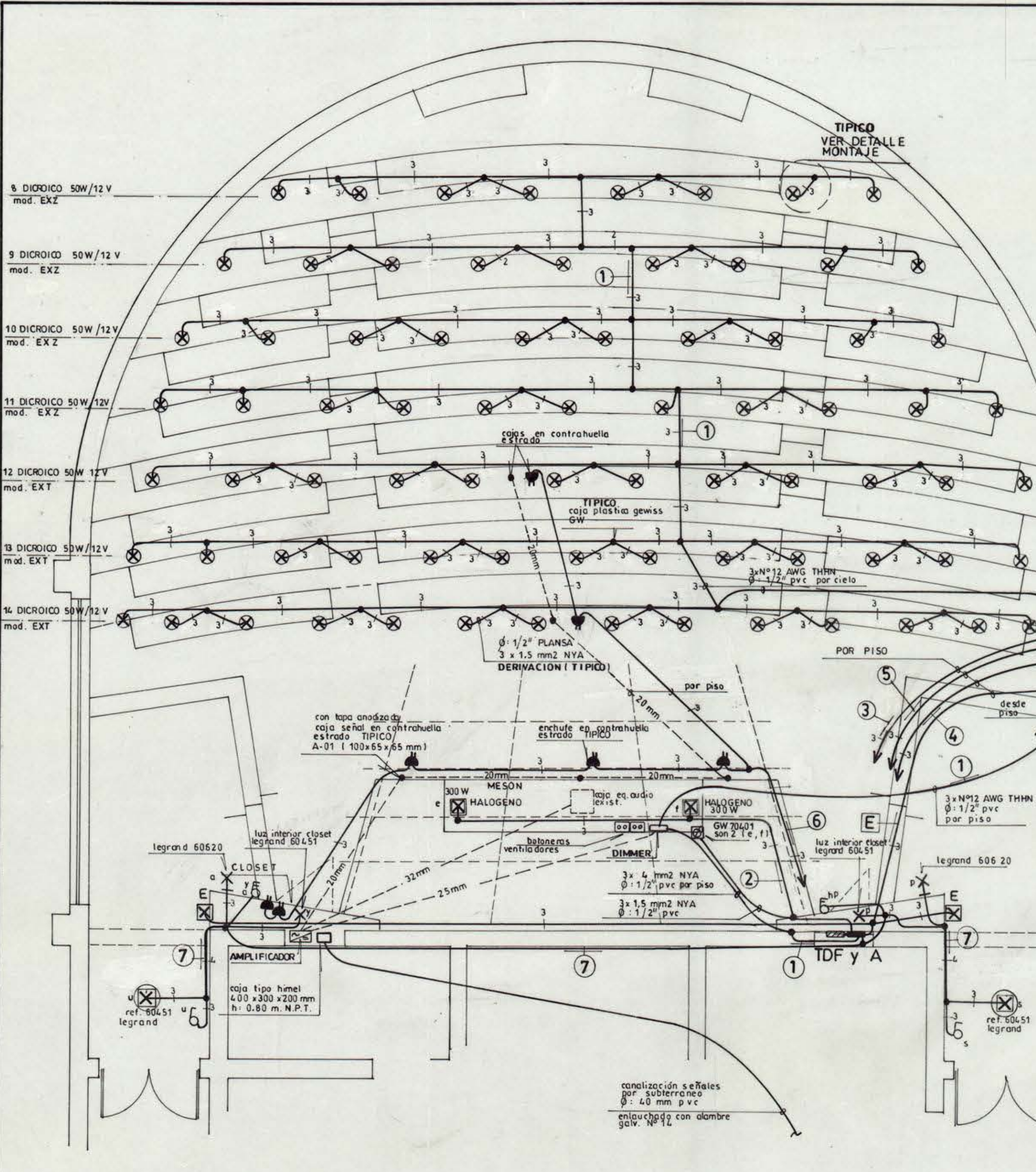
PLANTA AUDITORIUM Esc. 1:50
