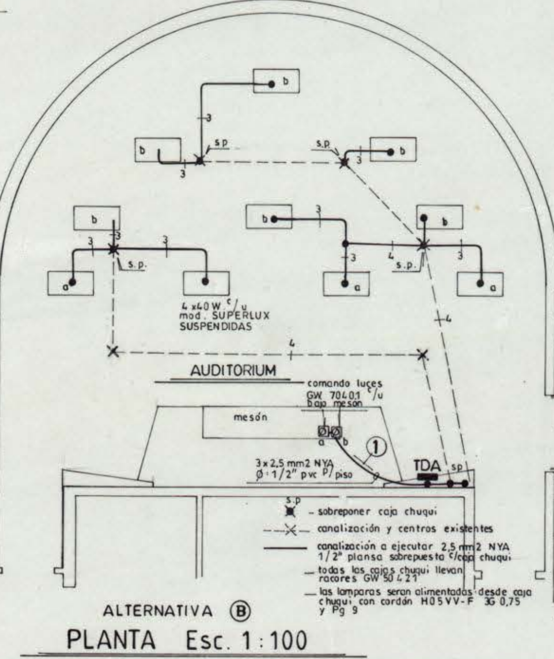
PLANTA Esc. 1:100
