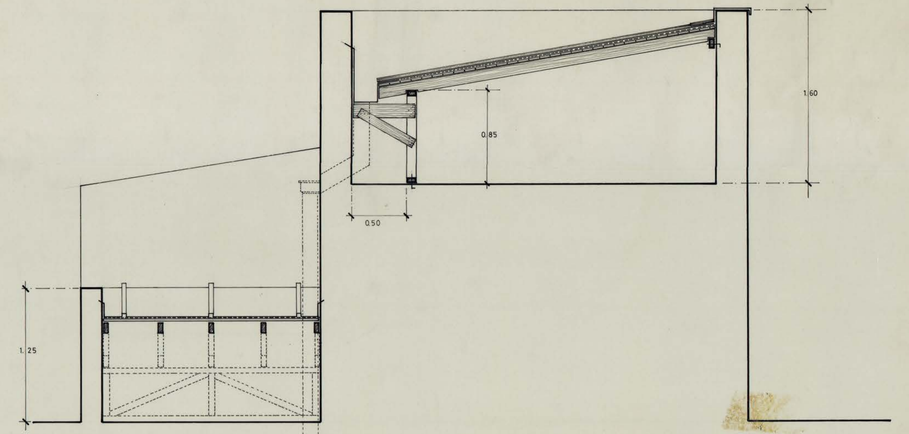
CORTE A - A ESC. 1:20
