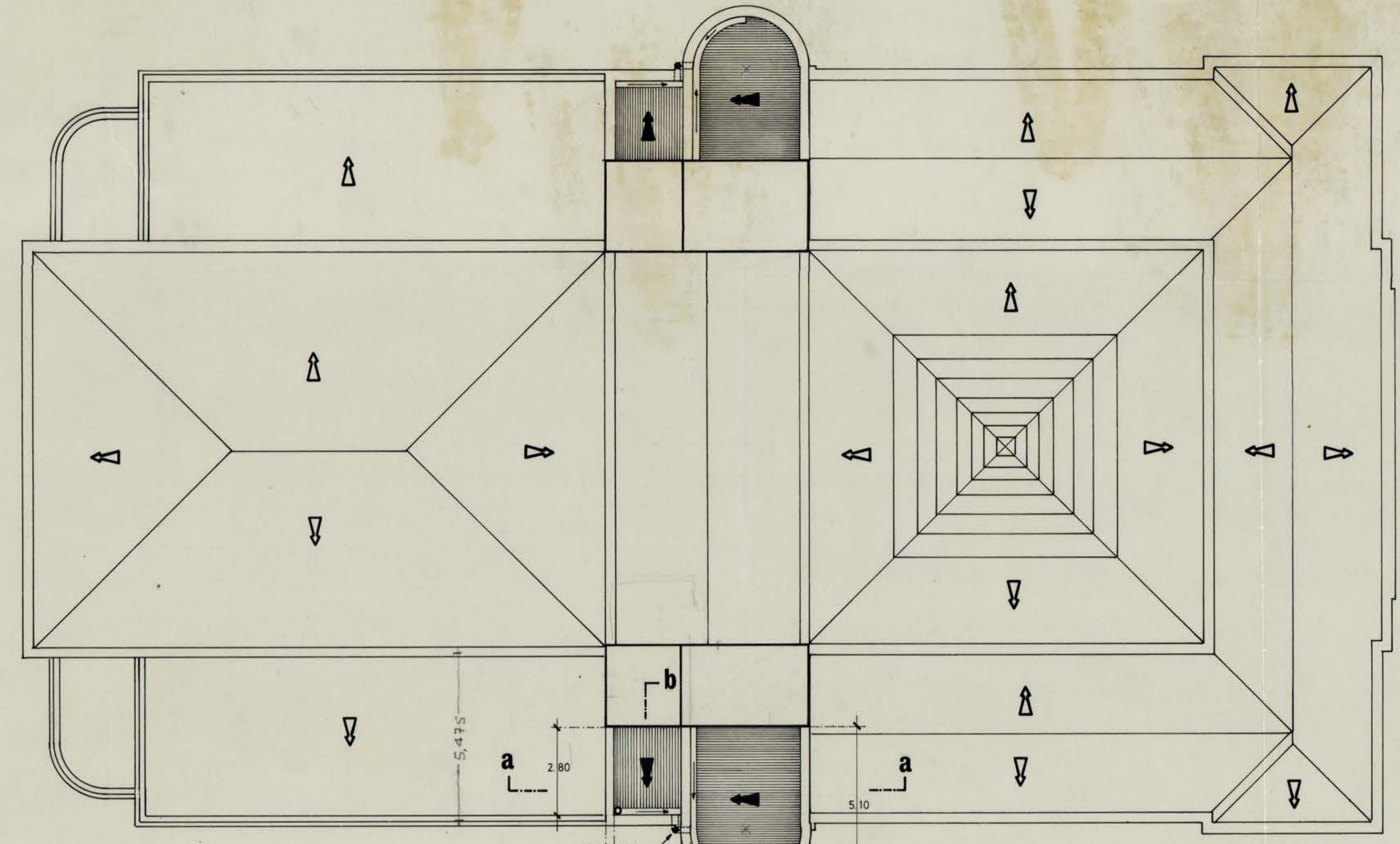
PLANTA TECHUMBRE ESC. 1:100
