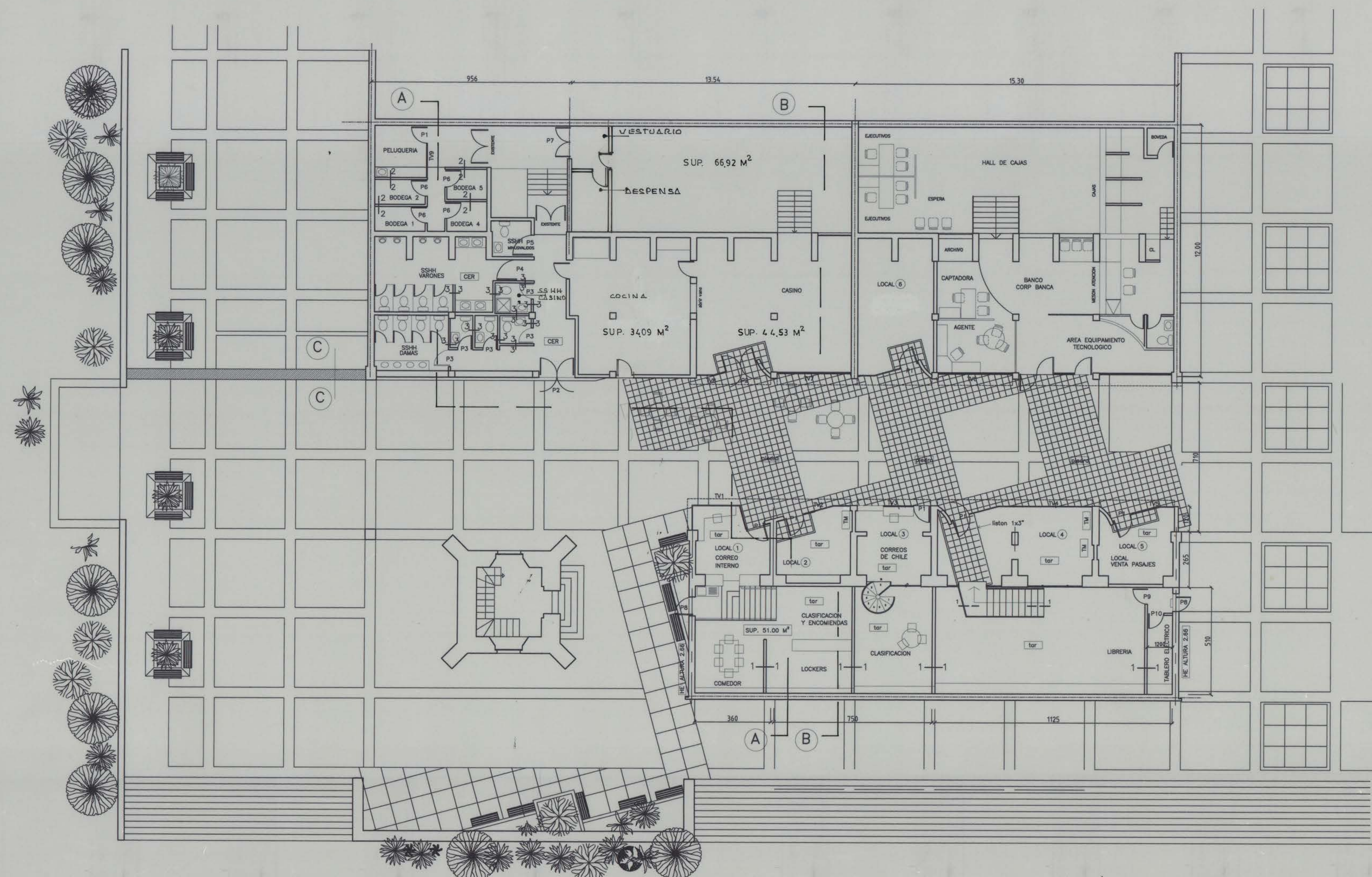
PLANTA ESC:1:100
