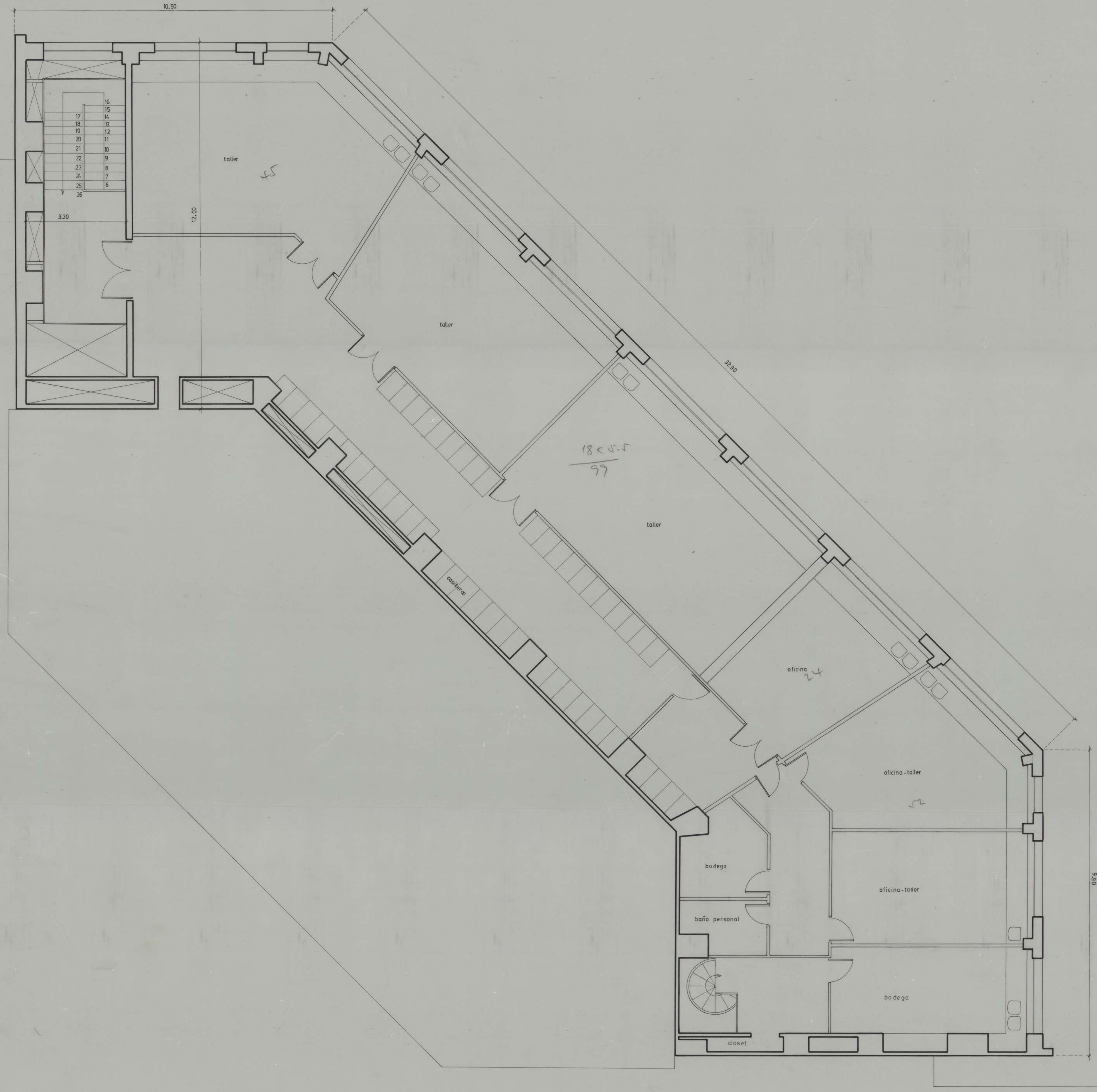
CASA DEL ARTE UNIVERSIDAD DE CONCEPCION ALEJANDRO RODRIGUEZ U. OSVALDO CACERES G. PLANTA TERCER PISO ESCALA 1:50
