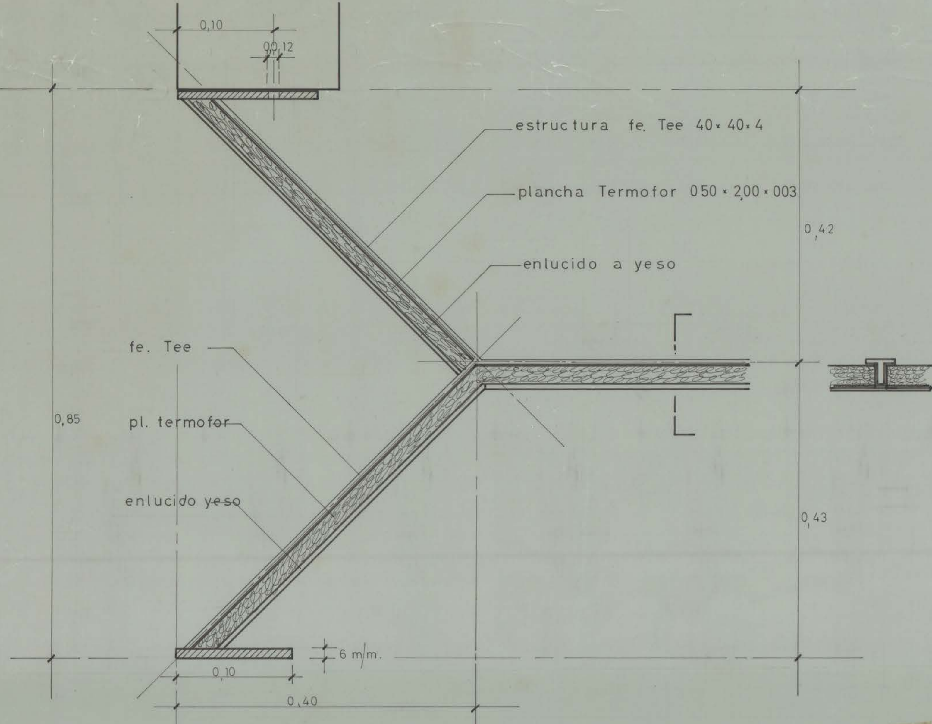
DETALLE CANAL CIELO FALSO escala 1:3
