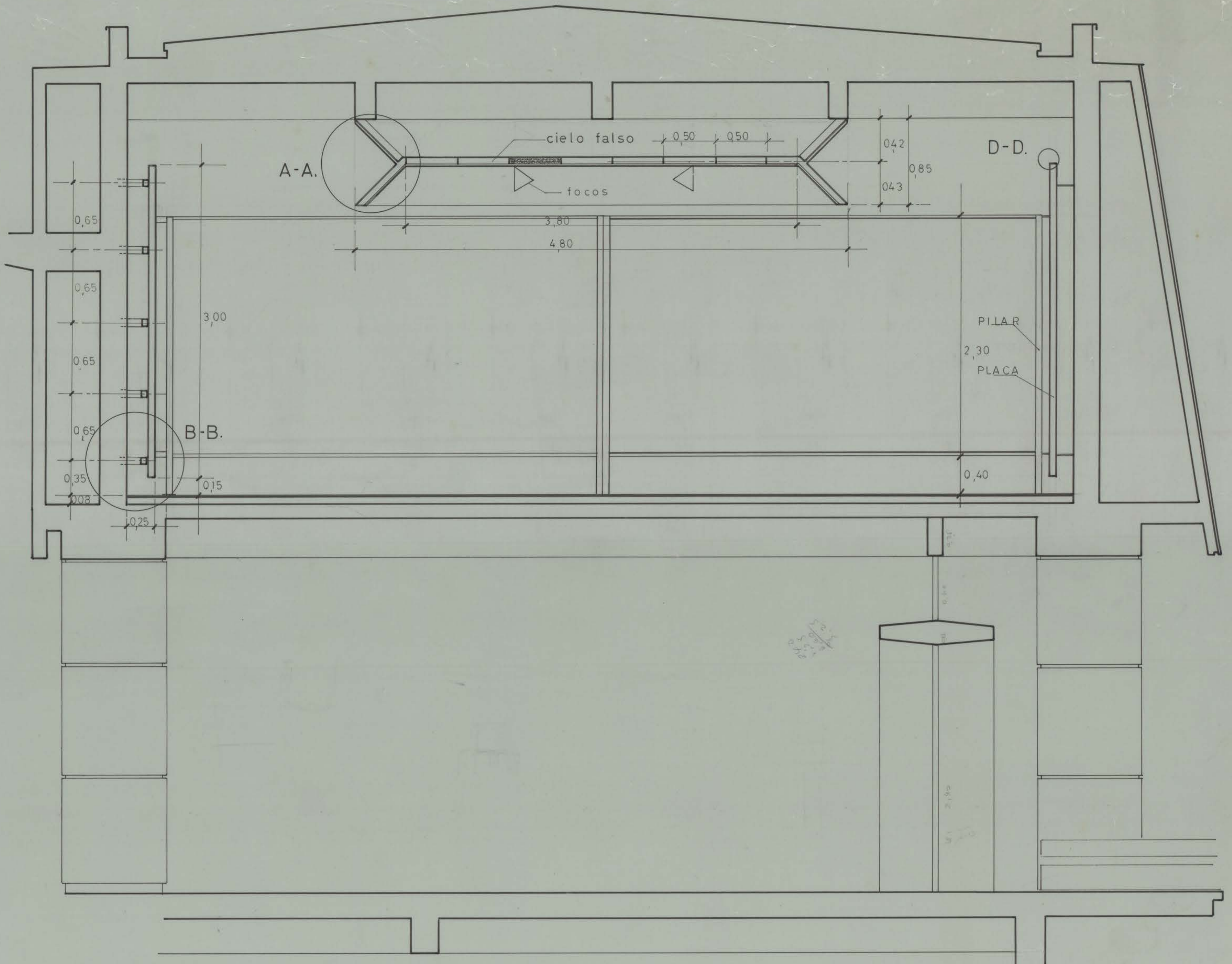
ELEVACION EN CORTE escala 1:20
