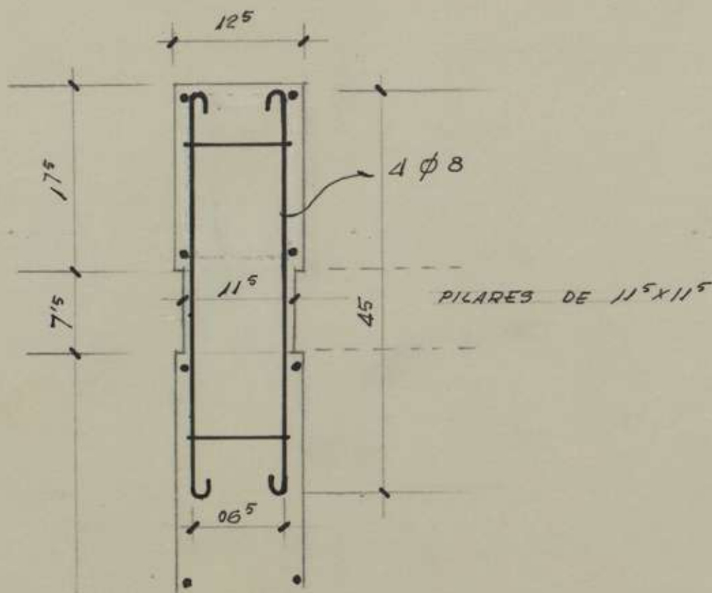
ARMADURA EN PILARES.
