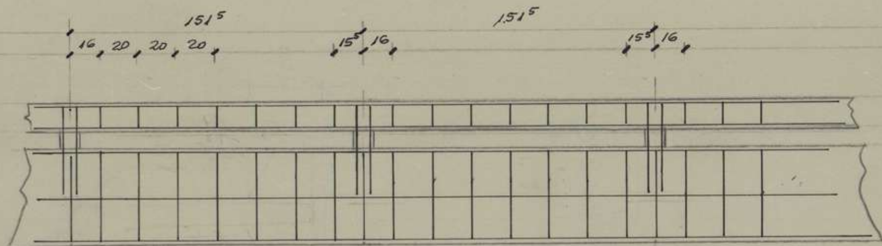
PILARES DE 115x115 CADA 1515 mts.
