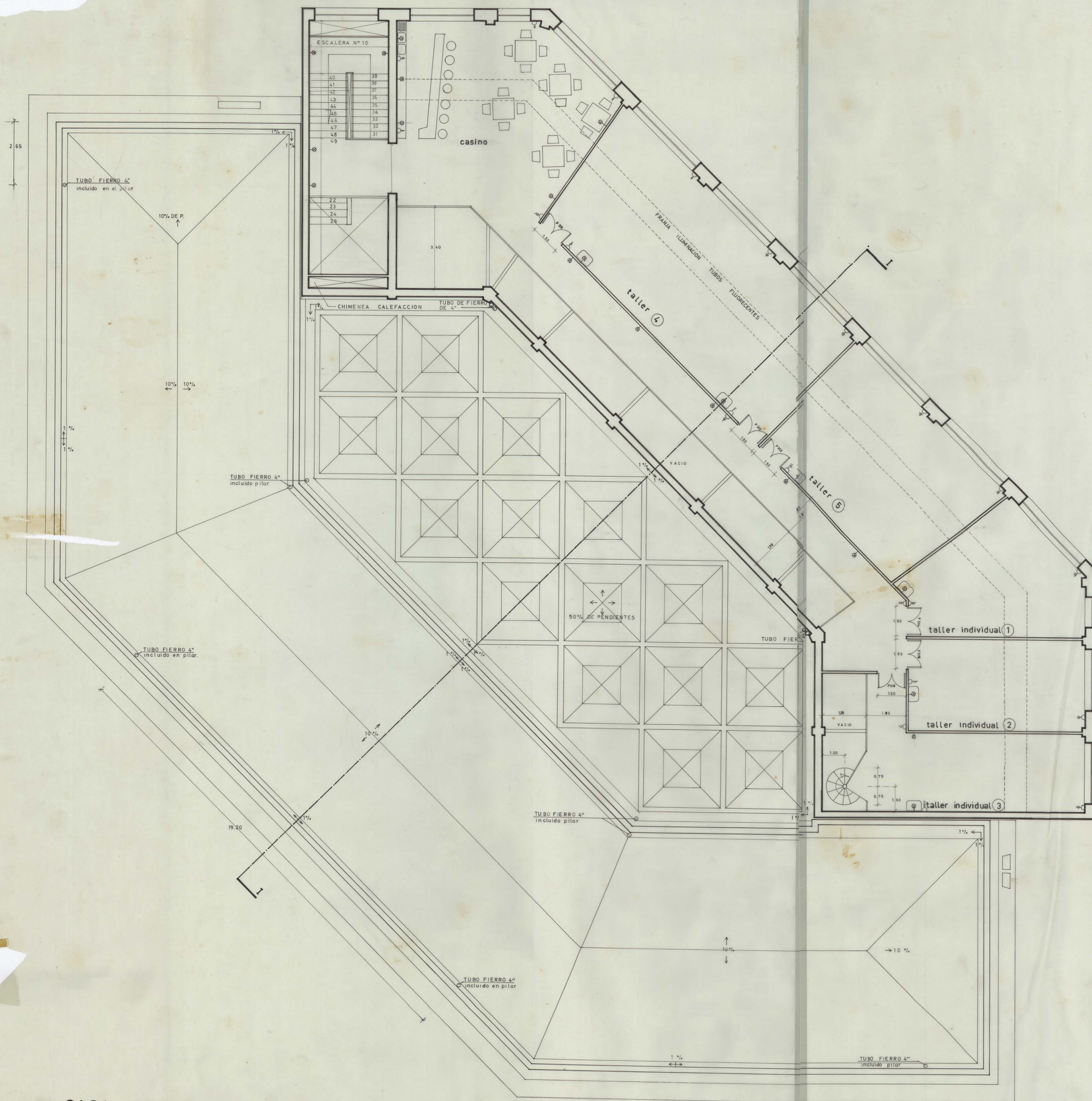
CASA DEL ARTE - UNIVERSIDAD DE CONCEPCION ARQUITECTOS ALEJANDRO RODRIGUEZ U. OSVALDO CACERES G. PLANTA TERCER PISO - ESCALA 1:50
