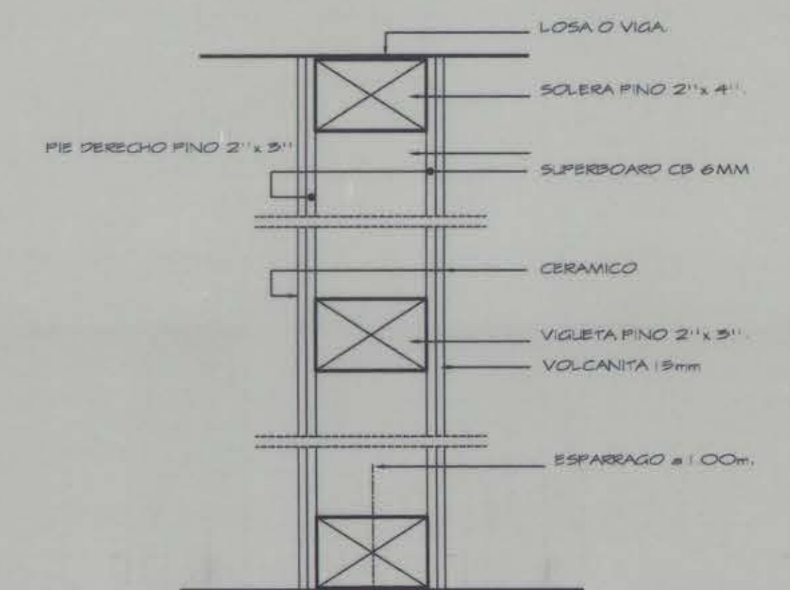
CORTE TABIQUE 3-3
