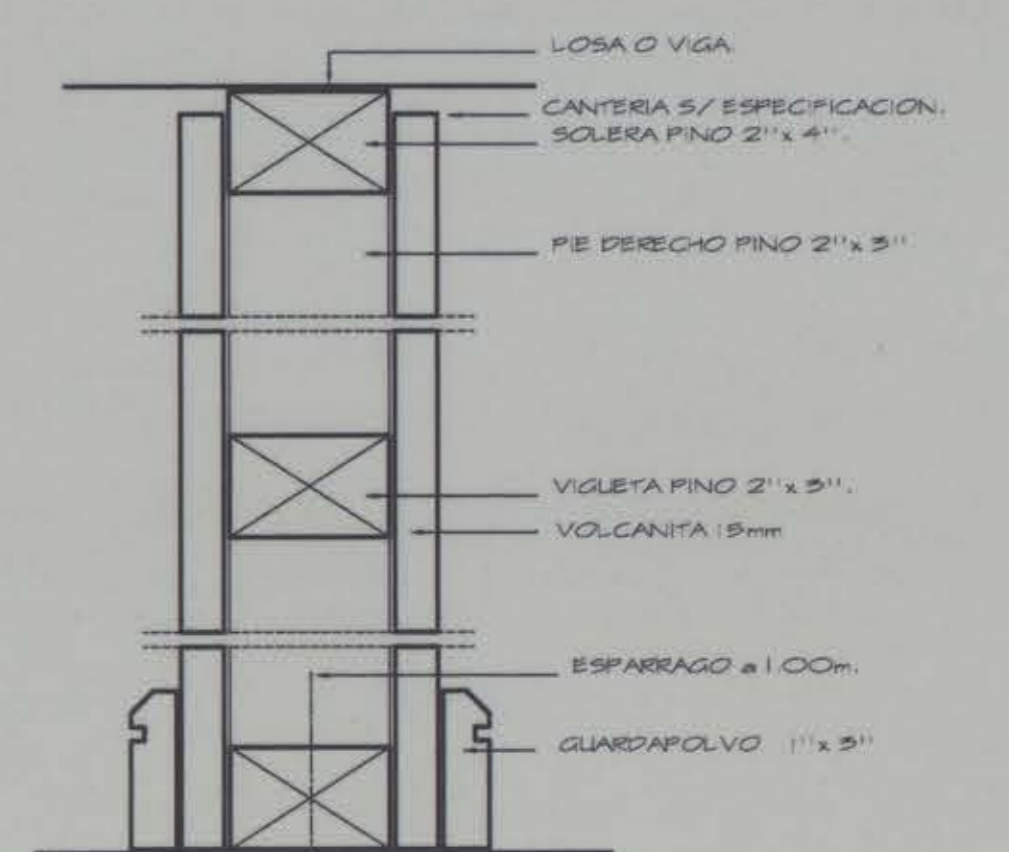
CORTE TABIQUE 2-2
