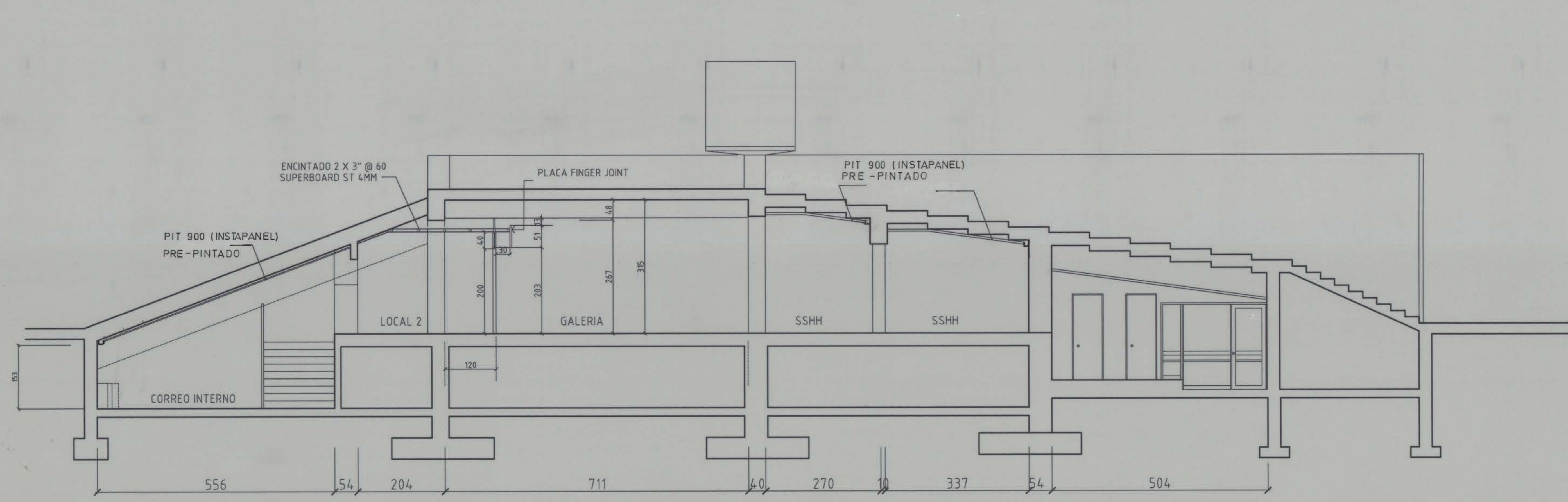
CORTE A-A
