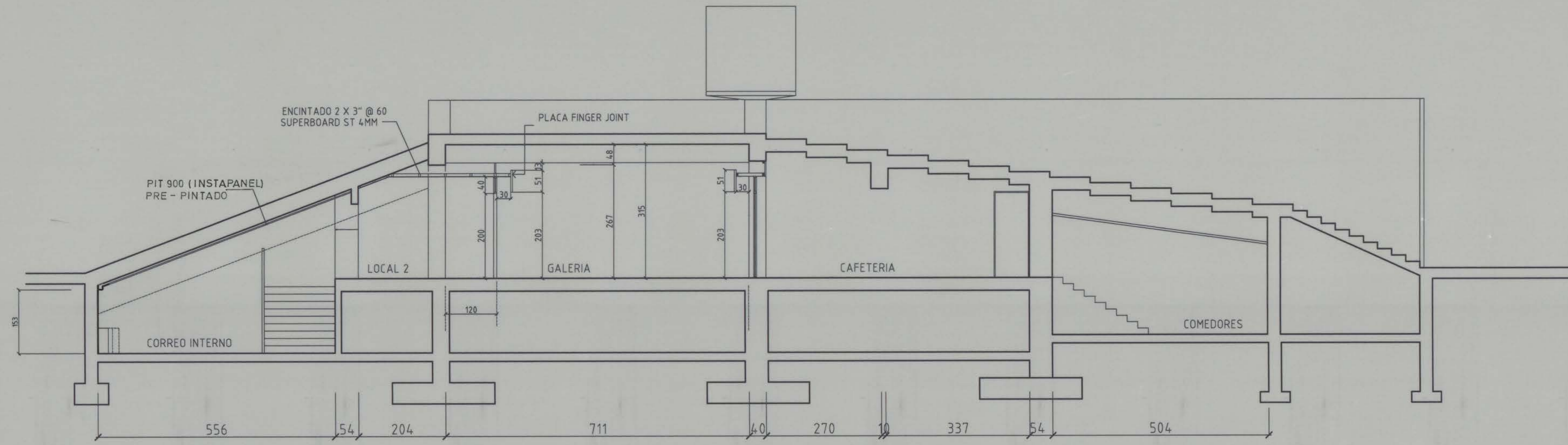
CORTE B-B
