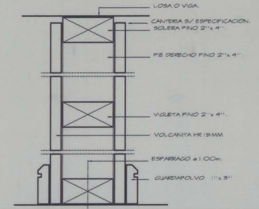
CORTE TABIQUE 1-1
