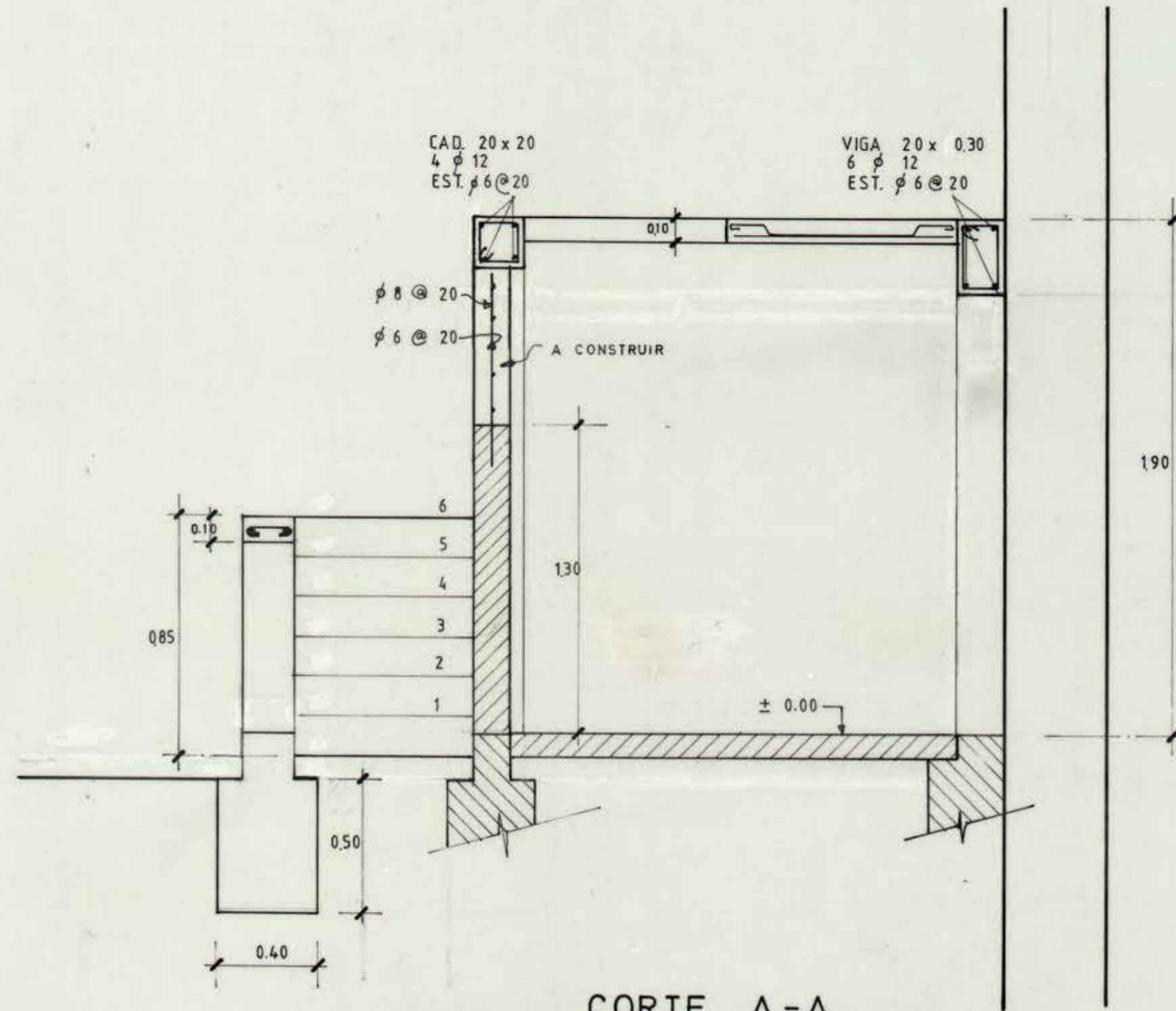
CORTE A-A
