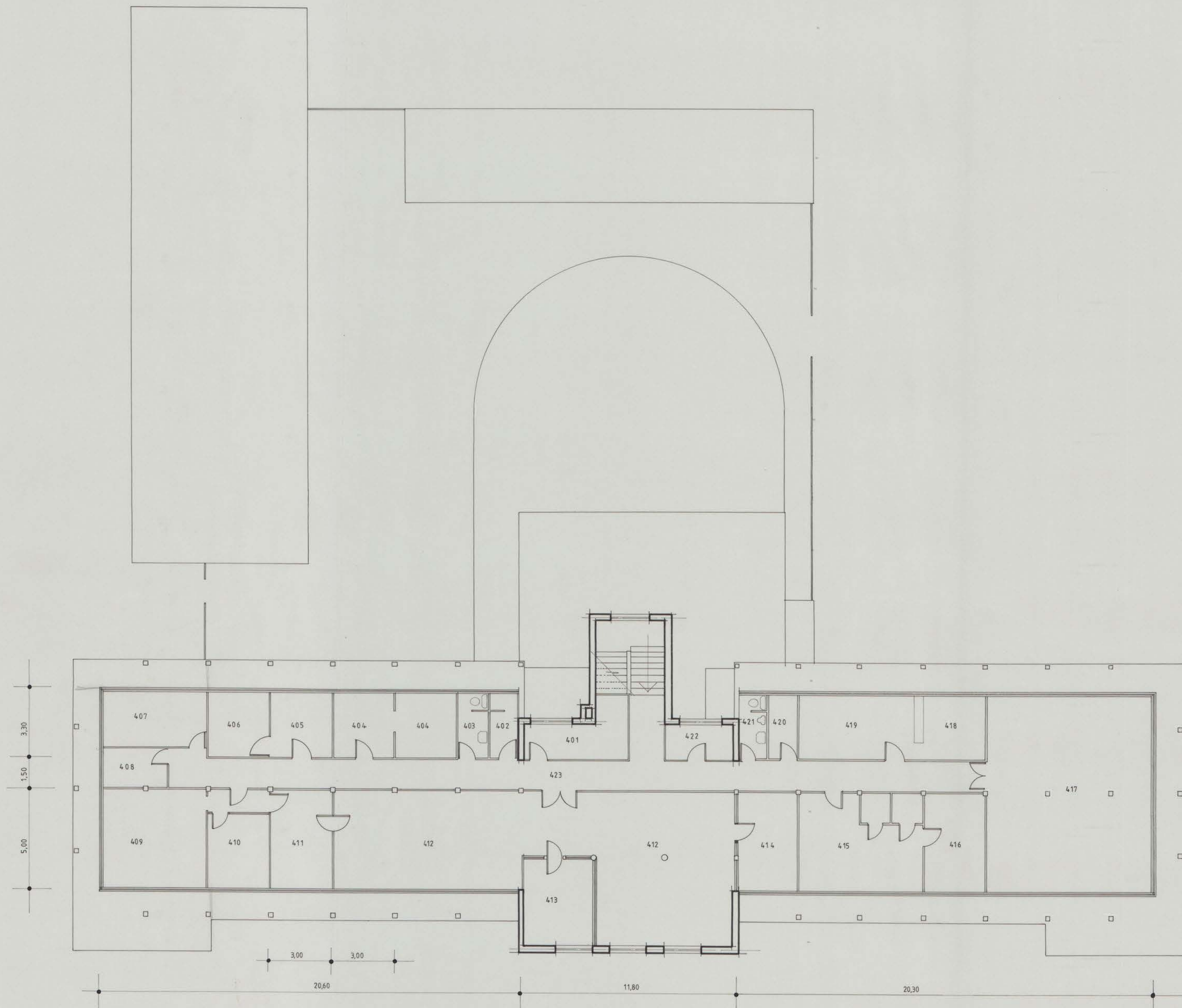
PLANTA 4to PISO EIDIFICIO DE BIOLOGIA
