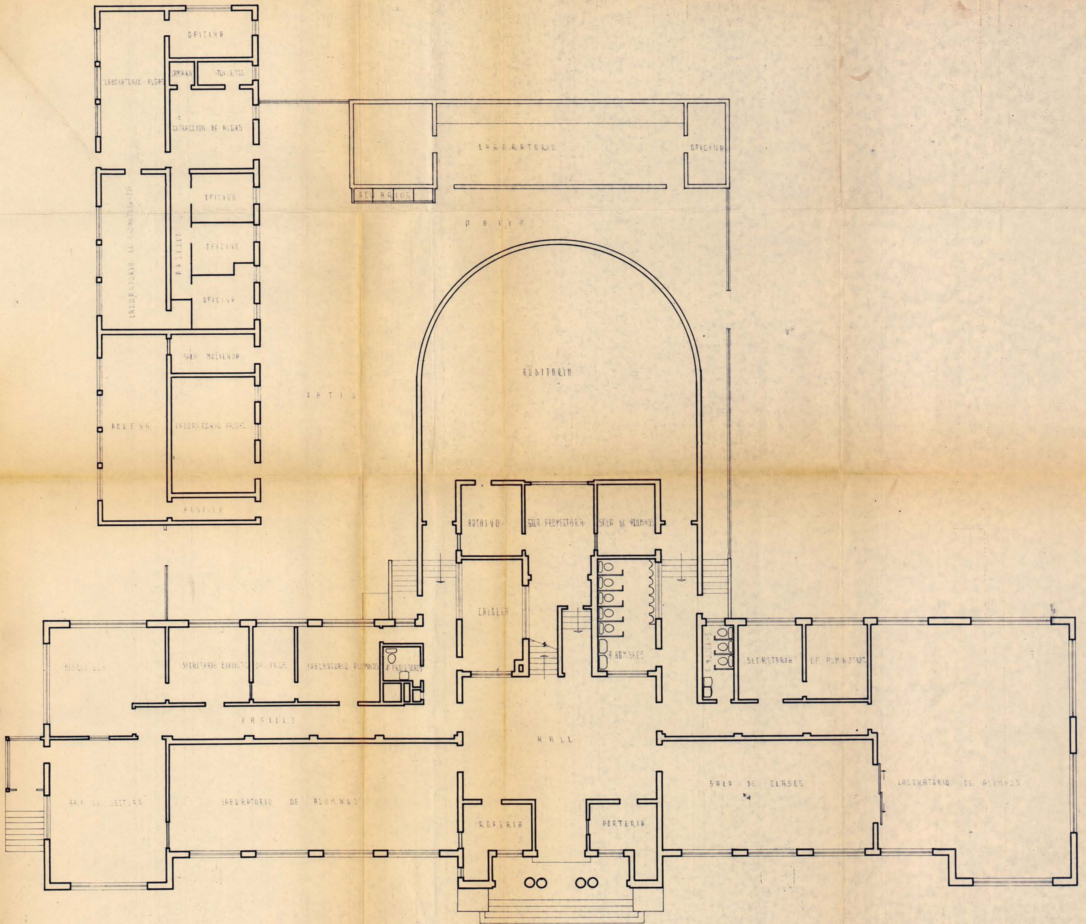
PLANTA PRIMER PISO Esc. 1 : 100
